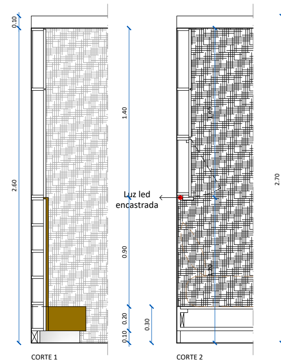
CORTE 1
