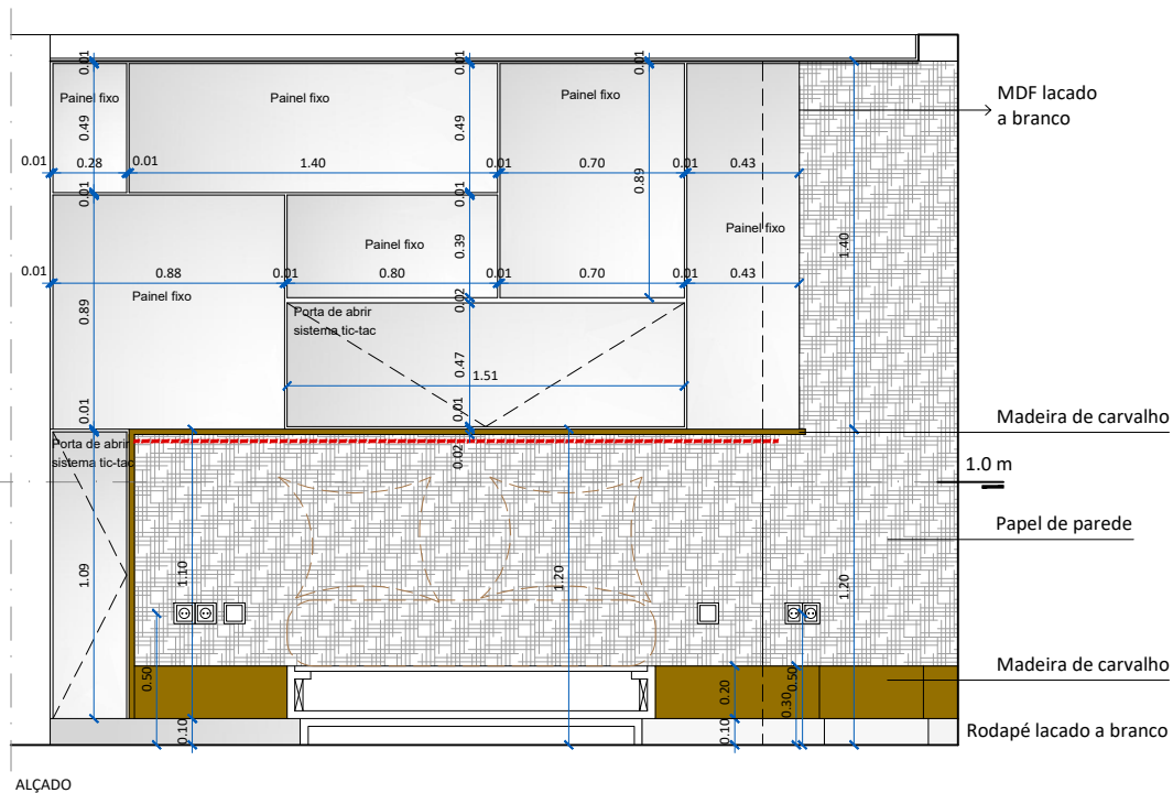
ALÇADO
